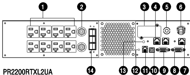
PR2200RTXL2UA
